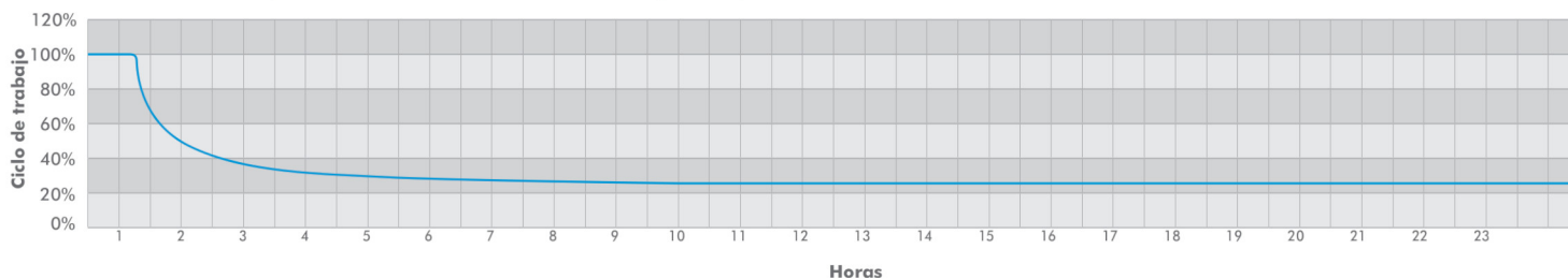
D5 SMART ciclo de trabajo de motor único en función del tiempo de operación
